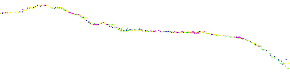
图 11 相邻航线以及相邻架次的点云数据的剖面图 程》NB/T 35109—2018 中对二级山地的点云数据高程中误差 1.340 m 的规定。该测区点云数据的绝对精度符合相关规范和技术设计要求,高程精度检查结果见表 2。点云数据高程中误差的分布基本满足正态分布,说明数据精度良好,没有出现整体性的系统误差。
