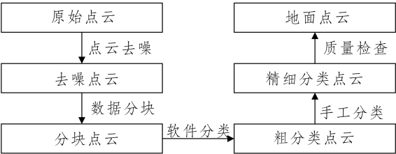
图 14 激光点云分类流程
