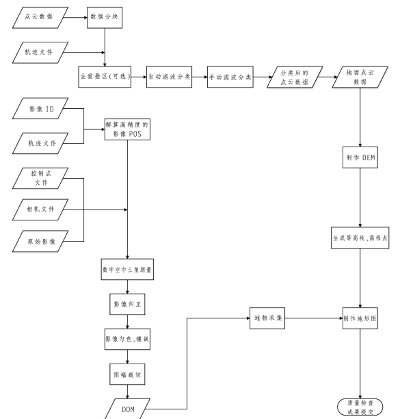
图 4 点云数据测绘产品生产流程图
