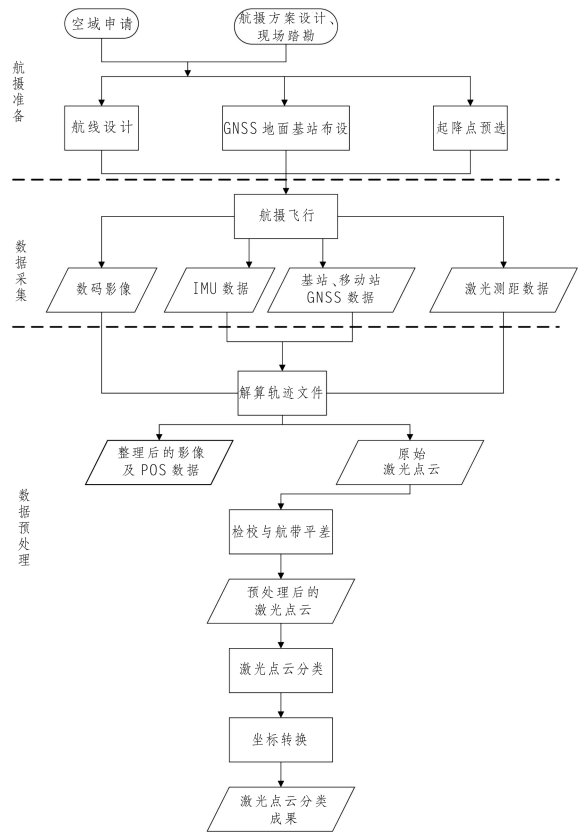
图 1 总体实施技术路线图
