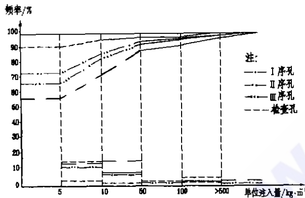
图1 挡水工程帷幕灌浆单位注入量频率曲线与频率累计曲线
