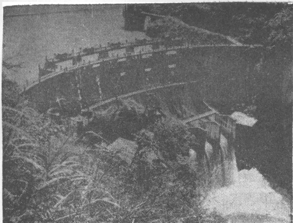
照片 4 四级窄巷口水电站 双拱坝侧视
