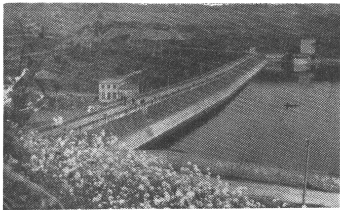
照片 1 一级红枫水电站 木斜墙堆石坝侧 视
