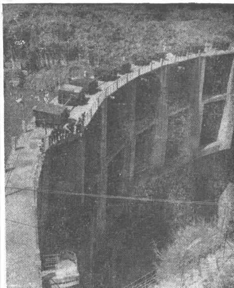
照片 6 b 双曲拱坝侧视
