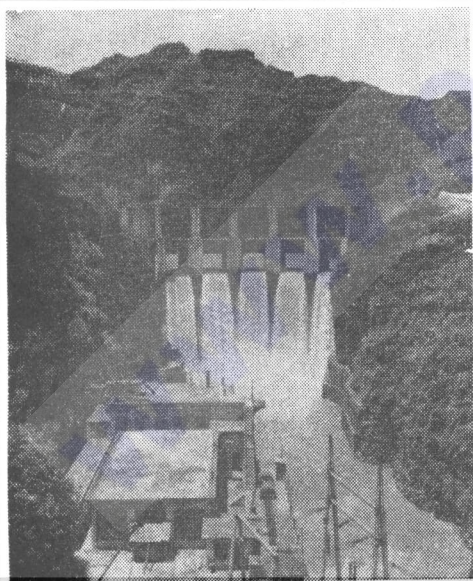
照片 6 a 六级红岩水电站双曲 拱坝下游上视
