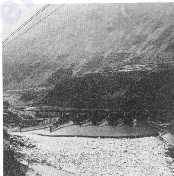
首部枢纽远景（左岸、下游上视）
