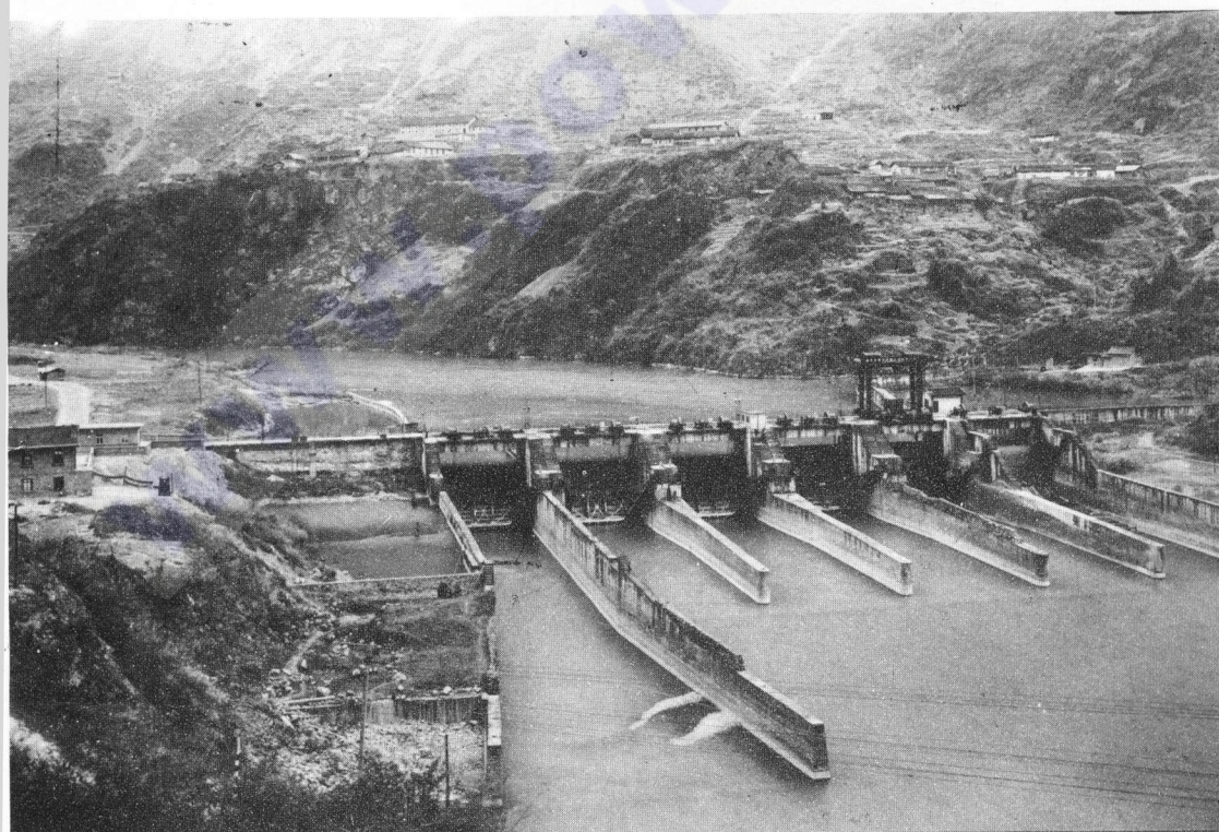
映秀湾水电站首部枢纽全景（二） （下游上视）
